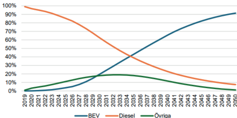
Figur 3: Andel tunga lastbilar (distributionstrafik) per drivmedel 2019-2050 14 . BEV står för Battery Electric Vehicle och är alltså de eldrivna lastbilarna.
